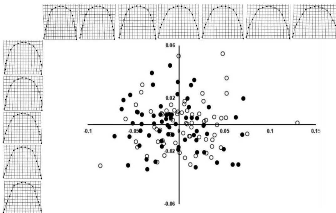
Figura 2: Variación de la forma según los componentes principales 1 y 2 (PC1= 50.14%, PC2= 13.31%). Las figuras muestran la variación antero-posterior del arco que ocurre en el eje horizontal o PC1. En el eje vertical (PC2) se aprecia la variación transversal del arco. Se observa claramente, además, la ausencia de diferencias respecto del sexo (mujeres en círculos blancos, hombres en círculos negros).
